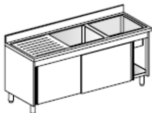
Lavatoio Su armadio, porte scorrevoli, 2 vasche, gocciolatoio sinistro
