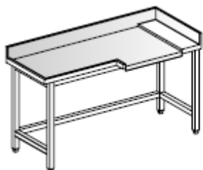
Tavolo uscita ad angolo con alzatina frontale e laterale, senza ripiano inferiore
