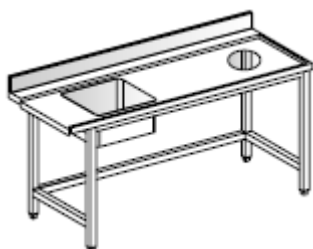
Tavolo entrata con alzatina e foro cernita , senza ripiano inferiore e vasca
