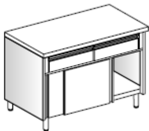
Tavolo armadio Porte scorrevoli, senza alzatina, con cassetti GN 1/1
